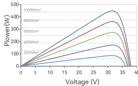
Power-Voltage(450W)
